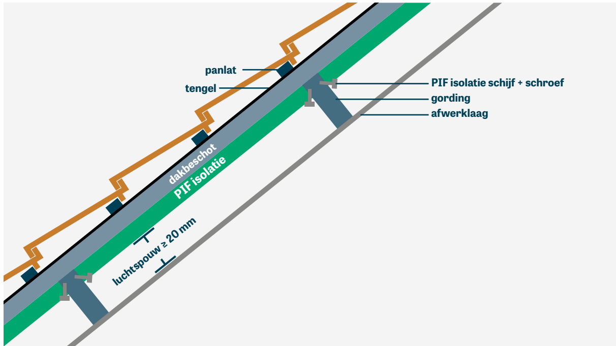
Bevestiging van PIF isolatie tegen dakbeschoot
